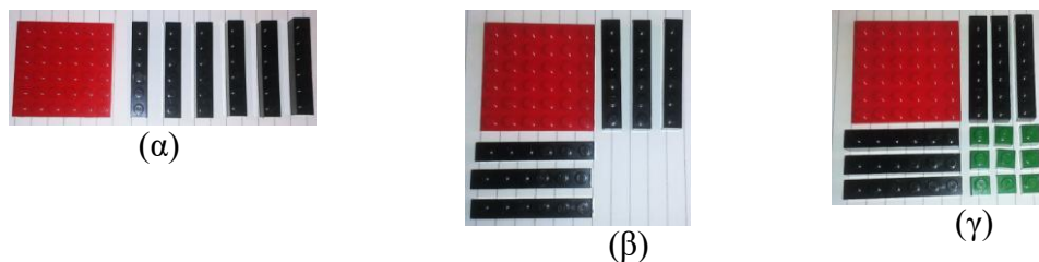
Σχήμα 4: Παράδειγμα μοντελοποίησης της τεχνικής της συμπλήρωσης τετραγώνου με Lego για εξισώσεις που είναι ή ανάγονται στη μορφή x^2 + 3x + c = 0
