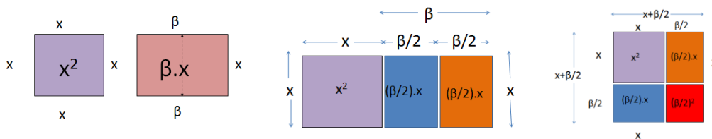
Σχήμα 6: Σχηματική αναπαράσταση της τεχνικής της συμπλήρωσης τετραγώνου γεωμετρικής επίλυσης της εξίσωσης x^2 + bx + \gamma = 0
