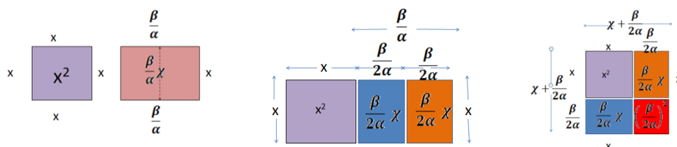
Σχήμα 7: Σχηματική αναπαράσταση της γεωμετρικής επίλυσης της εξίσωσης ax^2 + bx + \gamma = 0
