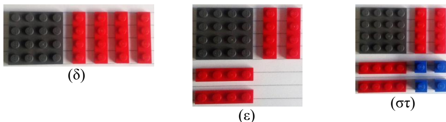
Σχήμα 5: Παράδειγμα μοντελοποίησης της τεχνικής της συμπλήρωσης τετραγώνου με Lego για εξισώσεις που είναι ή ανάγονται στη μορφή x^2 + 4x + c = 0
