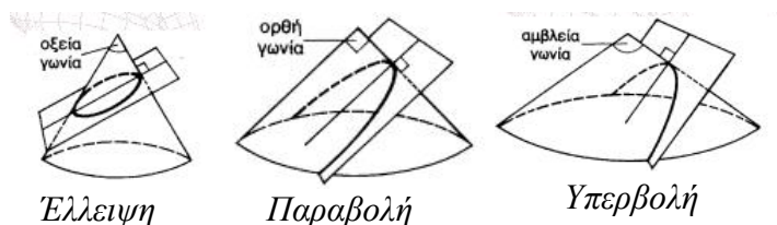
Σχήμα 1: Σχηματική αναπαράσταση των τριών κωνικών καμπυλών ως τομές κώνου – επιπέδου .
