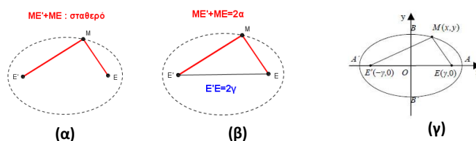
Σχήμα 3: (α), (β), (γ) Σχηματικές αναπαράσταση της έλλειψης σε ευκλείδειο και αναλυτικό επίπεδο
