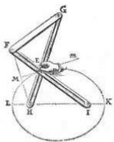
Σχήμα 8: Αναπαραστάσεις μοντέλου ελλειψογράφου του Frans van Schooten
