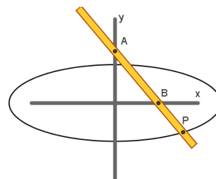
Σχήμα 7: Σχηματικές αναπαραστάσεις του ελλειψογράφου του Αρχιμήδη
