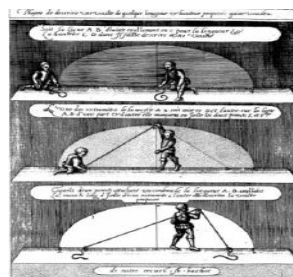
Σχήμα 6: Χρήση κορδονιού για το σχεδιασμό έλλειψης: Σχηματική (αριστερά) και εικονική αναπαράσταση (δεξιά) (Bachot, 1598 στο Barrallo et al., 2011)
