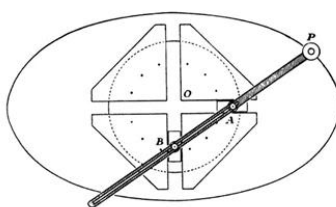
Σχήμα 7: Σχηματικές αναπαραστάσεις του ελλειψογράφου του Αρχιμήδη
