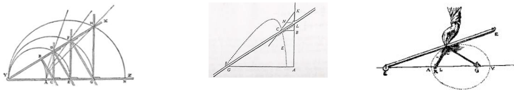
Σχήμα 5: Εργαλεία σχεδίασης καμπυλών από τον Descartes (Taimina et al., 2007)
