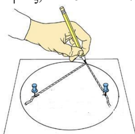
Σχήμα 6: Χρήση κορδονιού για το σχεδιασμό έλλειψης: Σχηματική (αριστερά) και εικονική αναπαράσταση (δεξιά) (Bachot, 1598 στο Barrallo et al., 2011)
