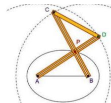
Σχήμα 8: Αναπαραστάσεις μοντέλου ελλειψογράφου του Frans van Schooten
